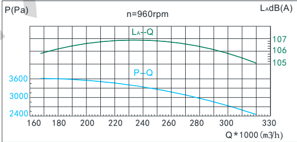
● Y4-73 20D性能曲线表
