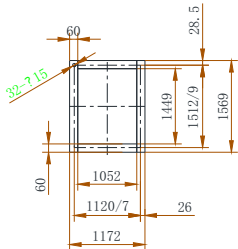
出风口联接尺寸
