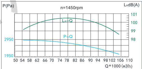
● Y4-73 12D性能曲线表
