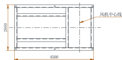
配台座基础尺寸
