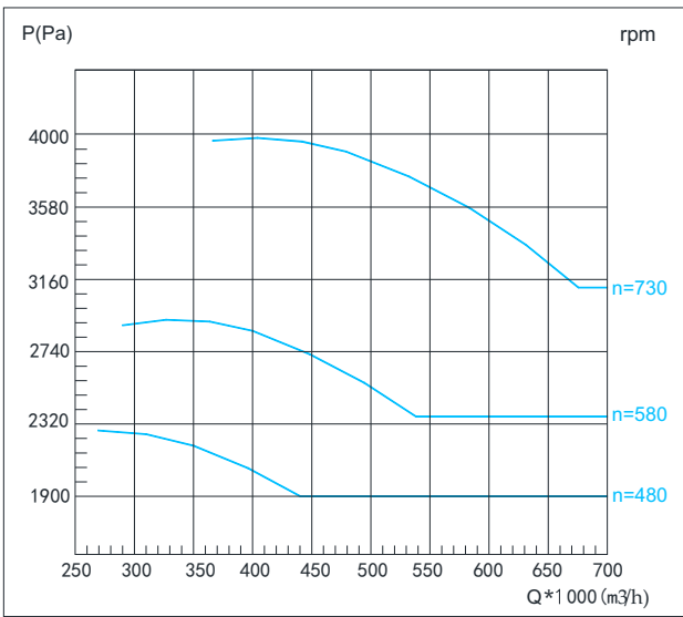
● Y4-73 28D性能曲线表
