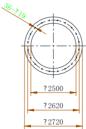
进风门联接尺寸
