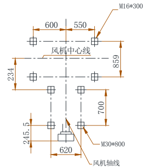
风机基础尺寸
