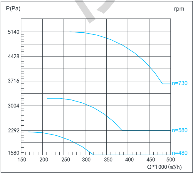
● G4-73 25D性能曲线表
