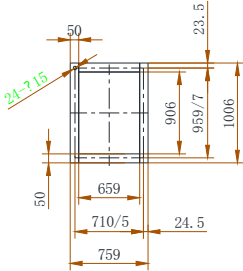
出风口联接尺寸
