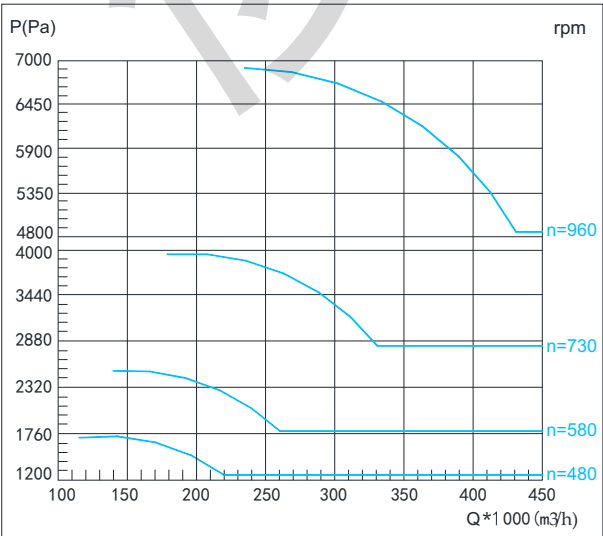
● G4-73 22D性能曲线表
