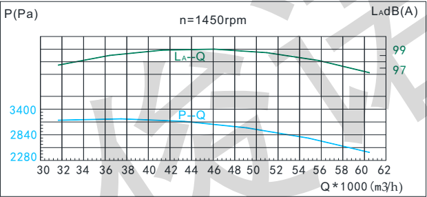
● G4-73 10D性能曲线表
