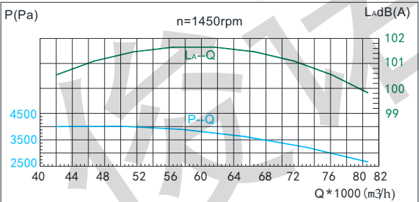
● G4-73 11D性能曲线表
