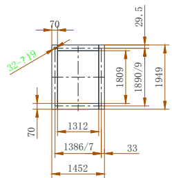
出风口联接尺寸
