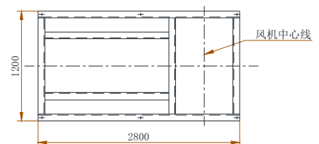
配台座基础尺寸
