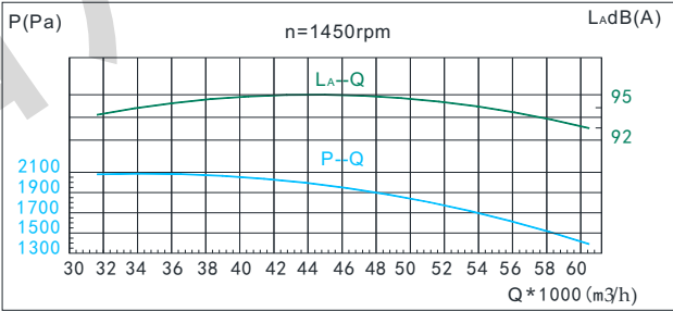
● Y4-73 10D性能曲线表
