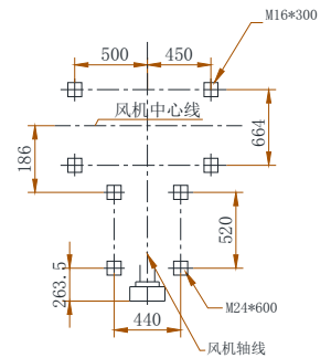
风机基础尺寸
