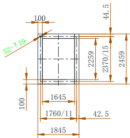
出风口联接尺寸
