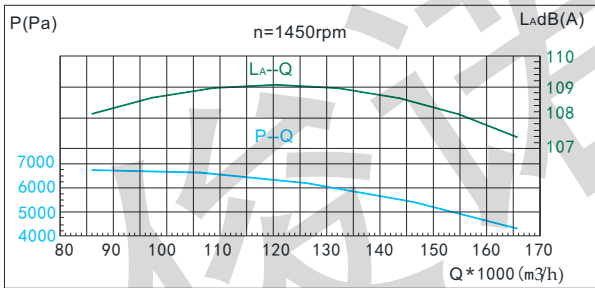
● G4-73 14D性能曲线表
