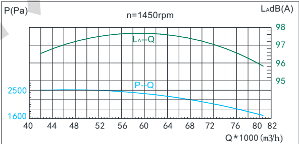
● Y4-73 11D性能曲线表
