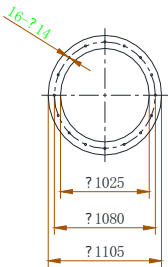
进风门联接尺寸
