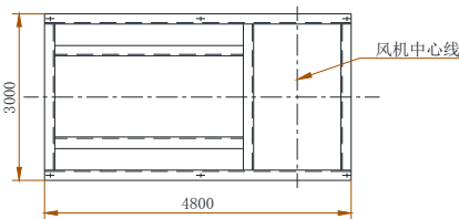
配套座基础尺寸
