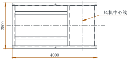
配台座基础尺寸
