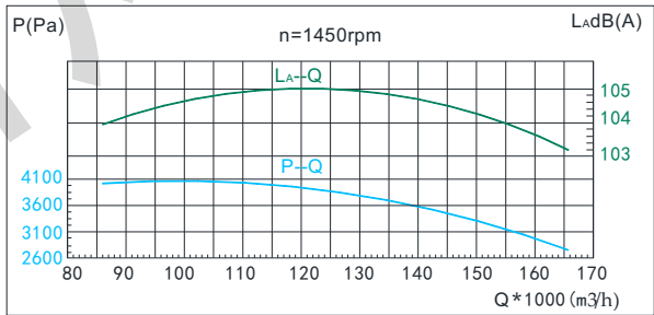
● Y4-73 14D性能曲线表
