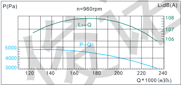
● G4-73 18D性能曲线表
