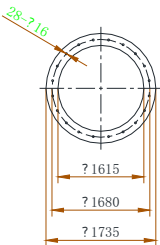
进风门联接尺寸
