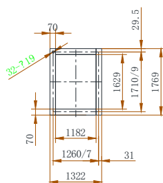
出风口联接尺寸
