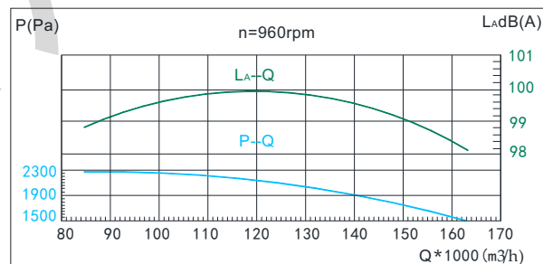
● Y4-73 16D性能曲线表
