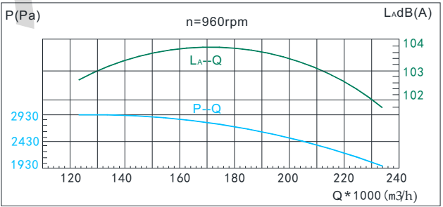
● Y4-73 18D性能曲线表
