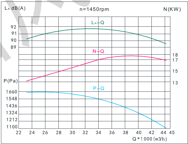
● Y4-73 9D性能曲线表
