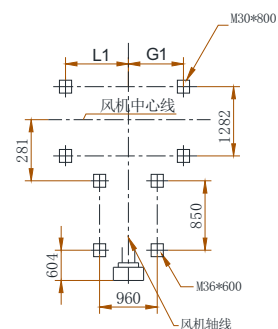
风机基础尺寸
