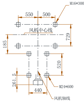
风机基础尺寸
