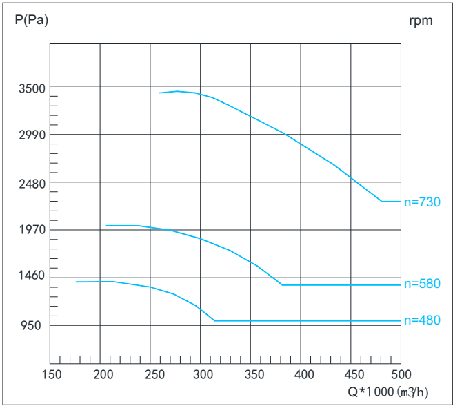
● Y4-73 25D性能曲线表
