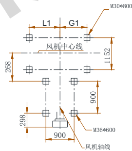
风机基础尺寸
