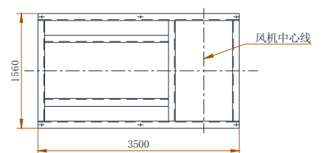
配台座基础尺寸
