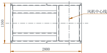
配台座基础尺寸
