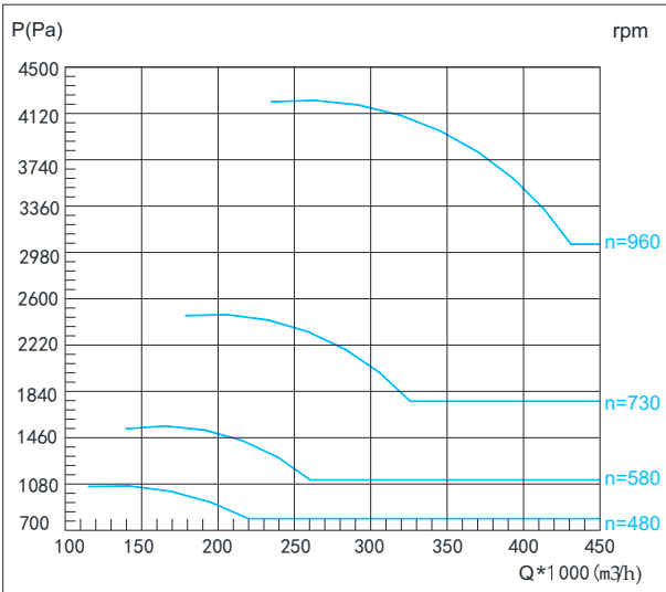
● Y4-73 22D性能曲线表
