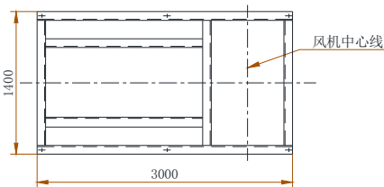
配套座基础尺寸
