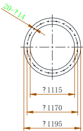
进风门联接尺寸
